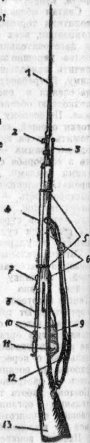
1—штык, 2—мушка с намушником, 3—шомпол, 4—ствольная накладка, 5—ложевые кольца, 6—ложа, 7—прицельная колодка, 8—ствольная коробка, 9—магазинная коробка, 10—затвор, 11—спусковой крючок, 12—ружейный ремень, 13—приклад.
